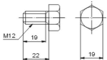
■ 卡具用螺栓 Bolts for Plate (CNS 2473之SS400或 CNS 3270之304) (SS 400 of CNS 2473 or 304 of CNS 3270)
