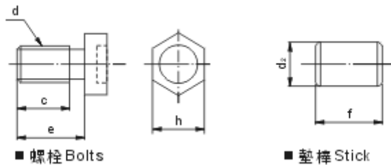
■ 螺栓 Bolts
