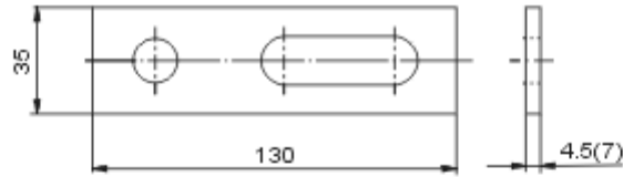
■ 卡具 Plate (CNS 2473之SS400或尼龍6) (SS 400 or nylon 6 of CNS 2473)
