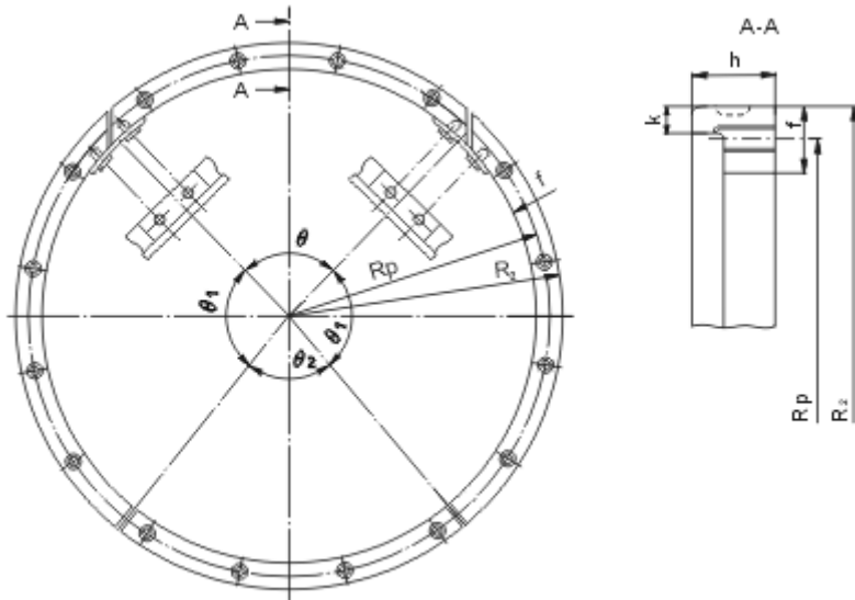
■ 壓圈 Gland
